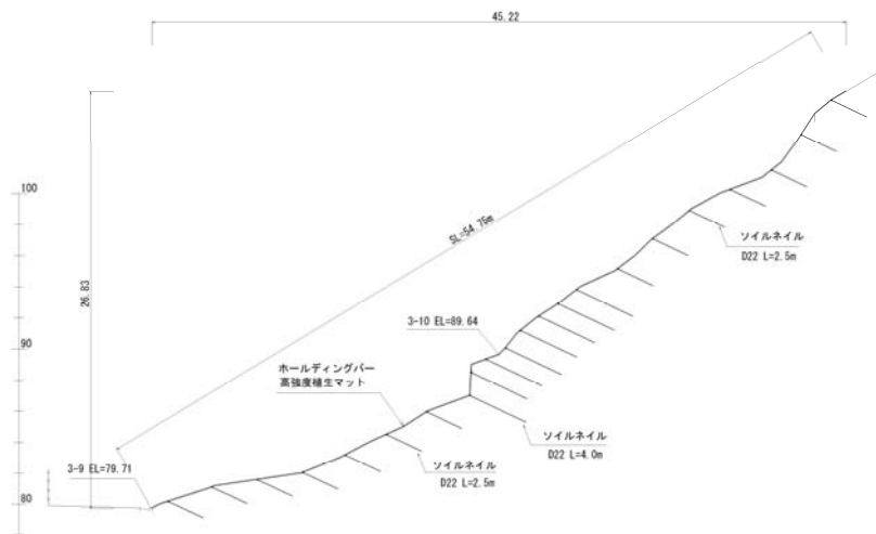
高強度植生マット、ベルトフレーム設置
